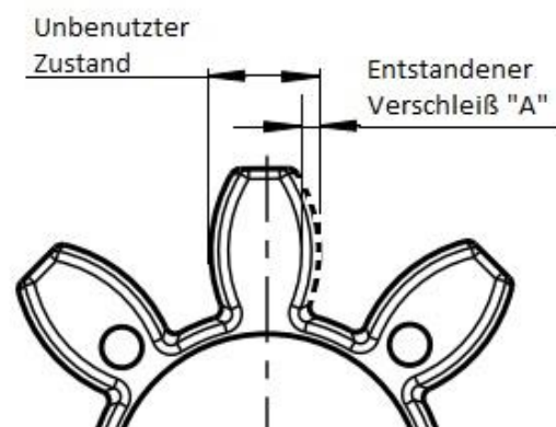
Abbildung 8: Verschleiß am Zahnkranz
